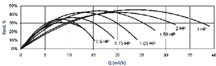
Curvas de rendimiento Performance curve
